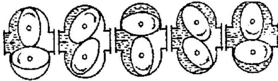
图1 椭圆齿轮运转原理图
