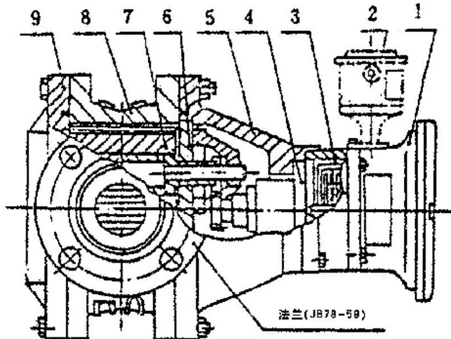
(图2) 椭圆齿轮流量计结构图
